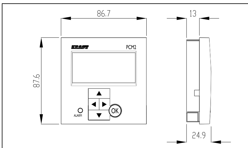
Måttskiss operatörspanel
