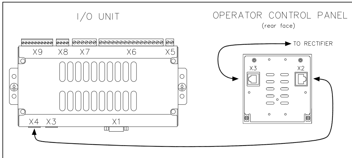
Anslutningar PCM2
