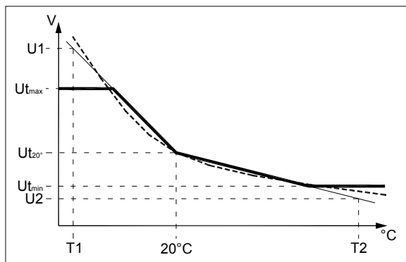
Figur 1: Temperaturkurva
