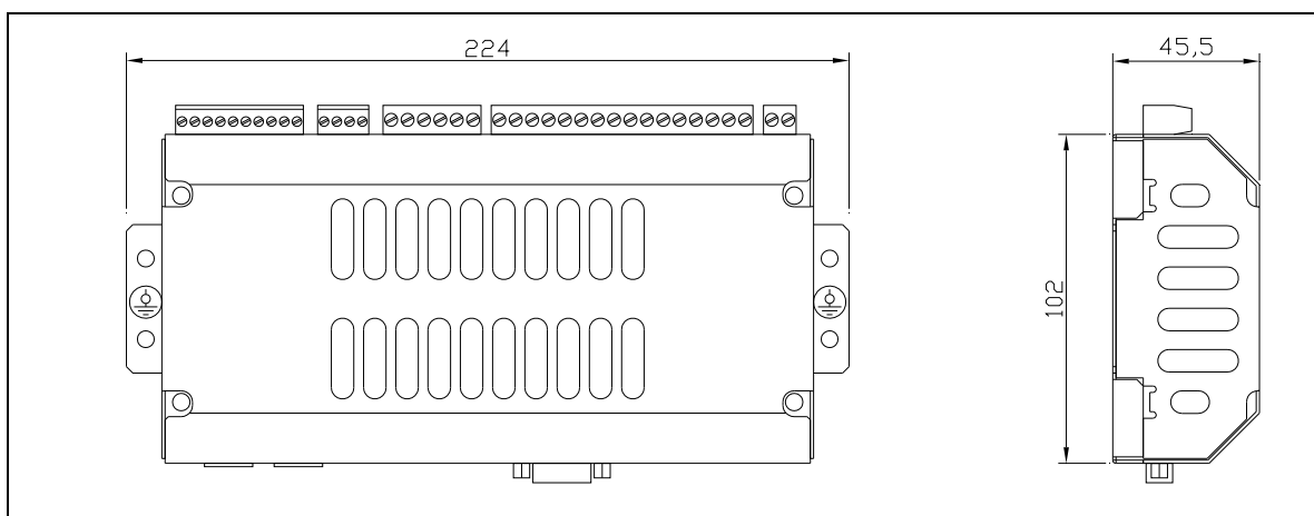
Måttskiss I/O-modul
